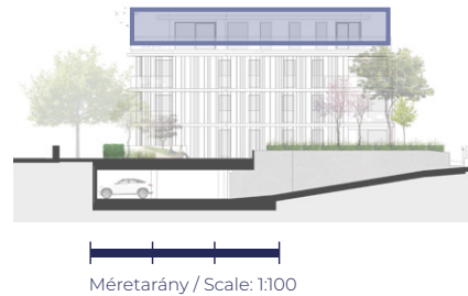
Metszet/ Section
