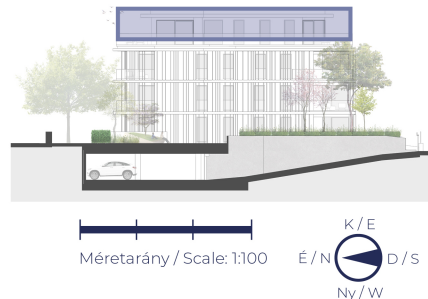
Metszet/ Section
