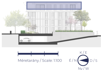
Metszet/ Section
